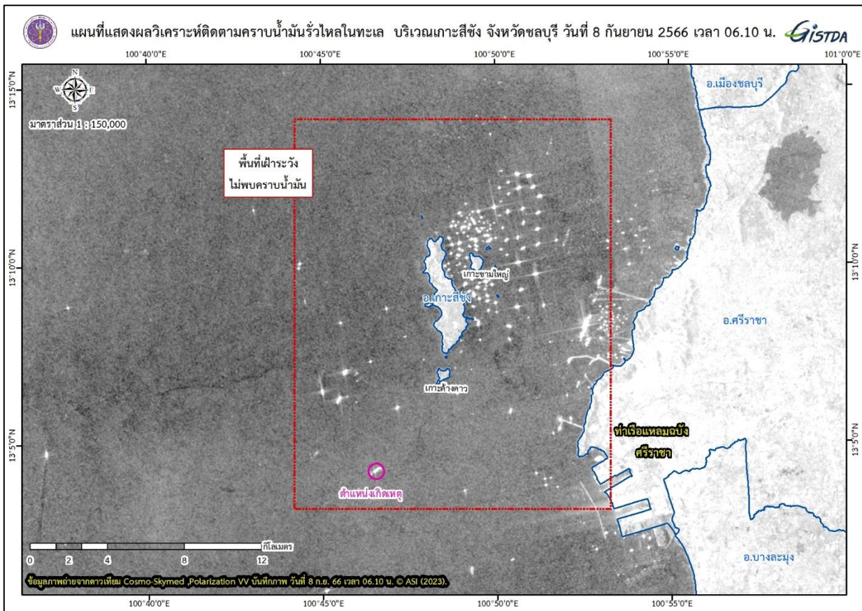
ภาพที่ 1 แผนที่แสดงผลวิเคราะห์ติดตามคราบน้ำมันในทะเล บริเวณเกาะสีชัง จังหวัดชลบุรี ภาพจากดาวเทียม COSMO-SkyMed วันที่ 8 กันยายน 2566 เวลา 06.10 น.
