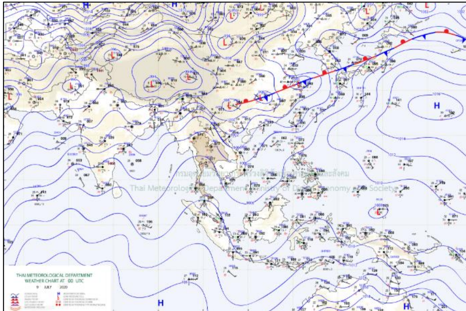
ภาพที่ 1 แผนที่อากาศผิวพื้นวันที่ 9 กรกฎาคม 2563 เวลา 07:00 น. มรสุมตะวันตกเฉียงใต้กำลังอ่อนพัดปกคลุมทะเลอันดามัน และประเทศไทย ในขณะที่มีลมใต้และลมตะวันออกเฉียงใต้พัดเข้ามาปกคลุมภาคตะวันออกเฉียงเหนือ ภาคตะวันออก และอ่าวไทย
